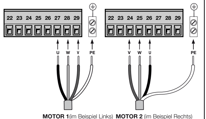
Anschluss an der Motorsteuerung MS1000
