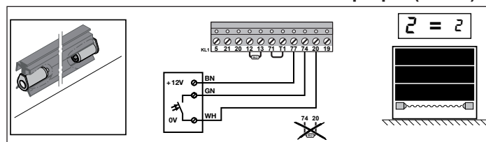
Capteurs optiques
