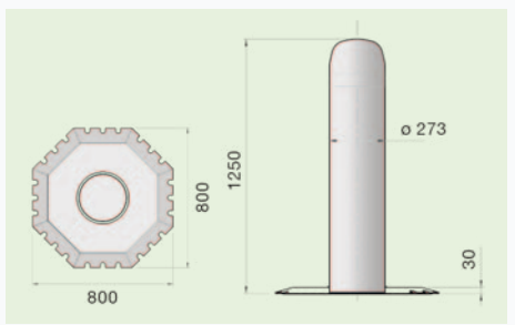
Abmessungen SafetyGuard 350/450TR (mm)
