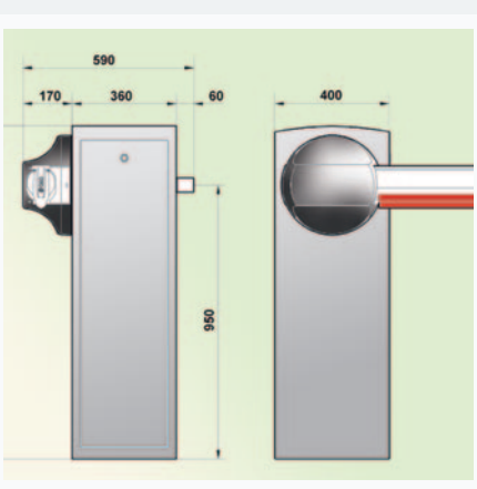
Abmessungen B6010 (mm)
