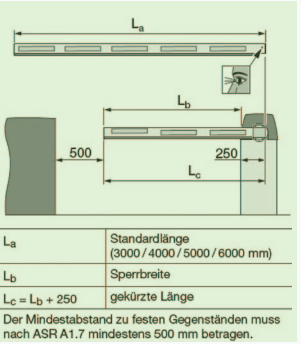
Torschranke BS60
