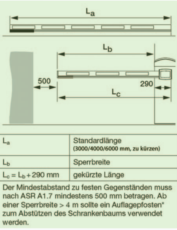
Torschranke BS50
