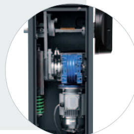
Stabile und robuste Mechanik
