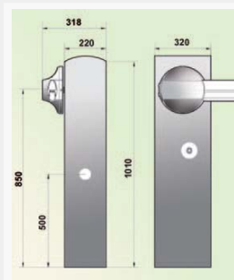
Dimensions B23/B24/B25 (mm)
