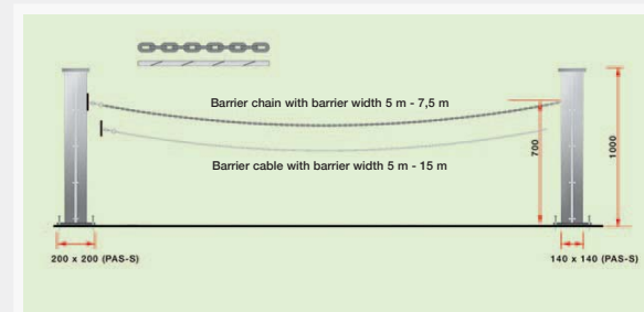
Absenker PAS mit Bodenplatte (mm)
