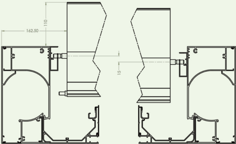
Lamellen in geöffneter Position
