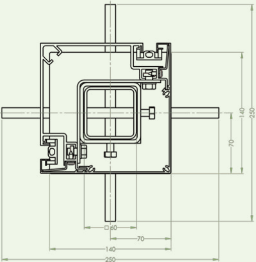
c. Befestigung über Bodenanker Einen Bodenanker mit einem Betonblock (Fundament) bereitstellen: 50 cm 50 cm x 100 cm (Tiefe)
