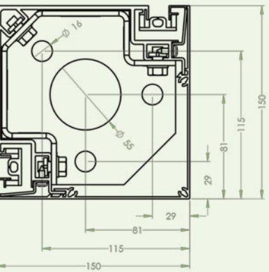
a. Standardbefestigung am Boden
