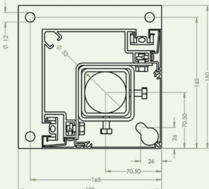
b. Befestigung über Bodenplatte
